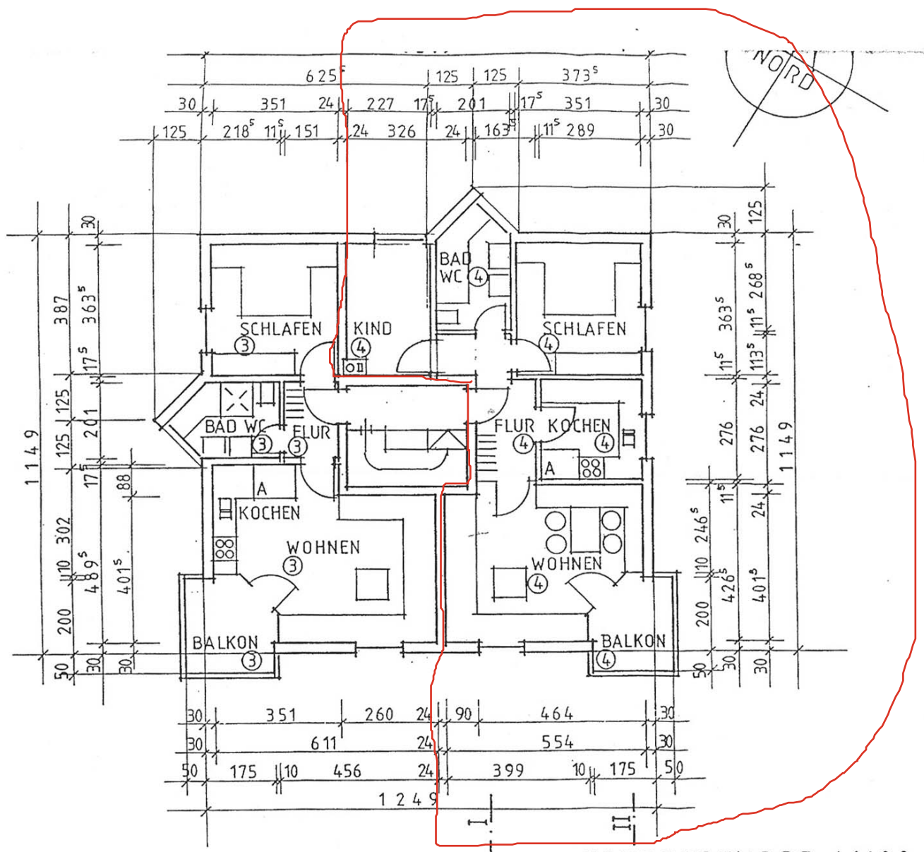
OBERGESCHOSS 1/100
